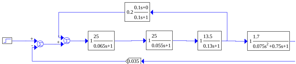
Рисунок 3.3– Исходный замкнутый контур (модель) объекта управления
