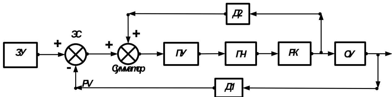
Рисунок 3.2 – Пример структурной схема САР
