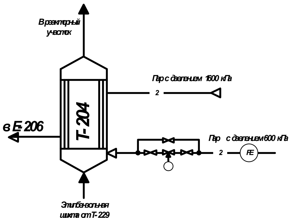
Рисунок 3.1 – Пример технологической схемы объекта
